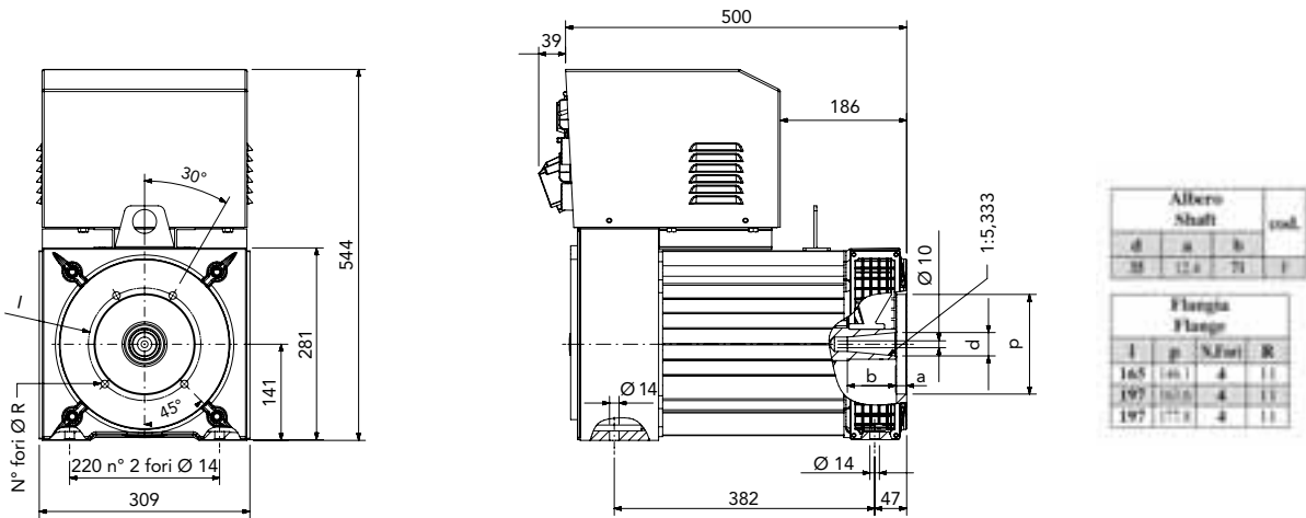
Forma costruttiva / Shape IM B35 - J609b cod. F
