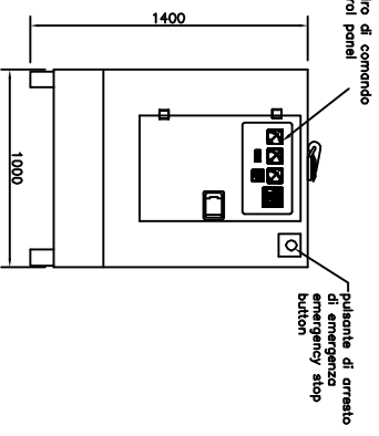
VISTA LATO ALTERNATORE ALTERNATOR SIDE VIEW
