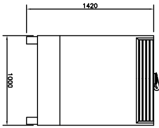
VISTA LATO MOTORE ENGINE SIDE VIEW
